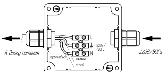
Схема подключения.
