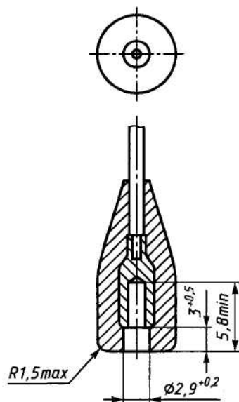
Рисунок 1 - Пример приемлемого соединения для гирлянды
